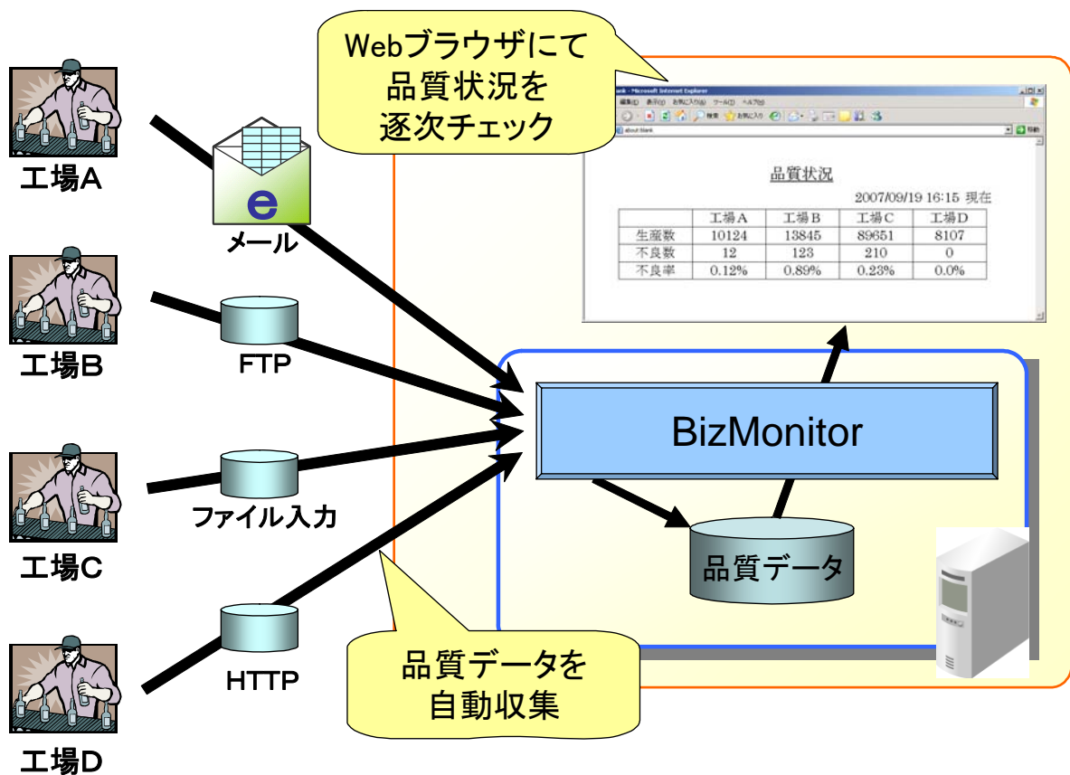
BizMonitor によるシステム構成例
